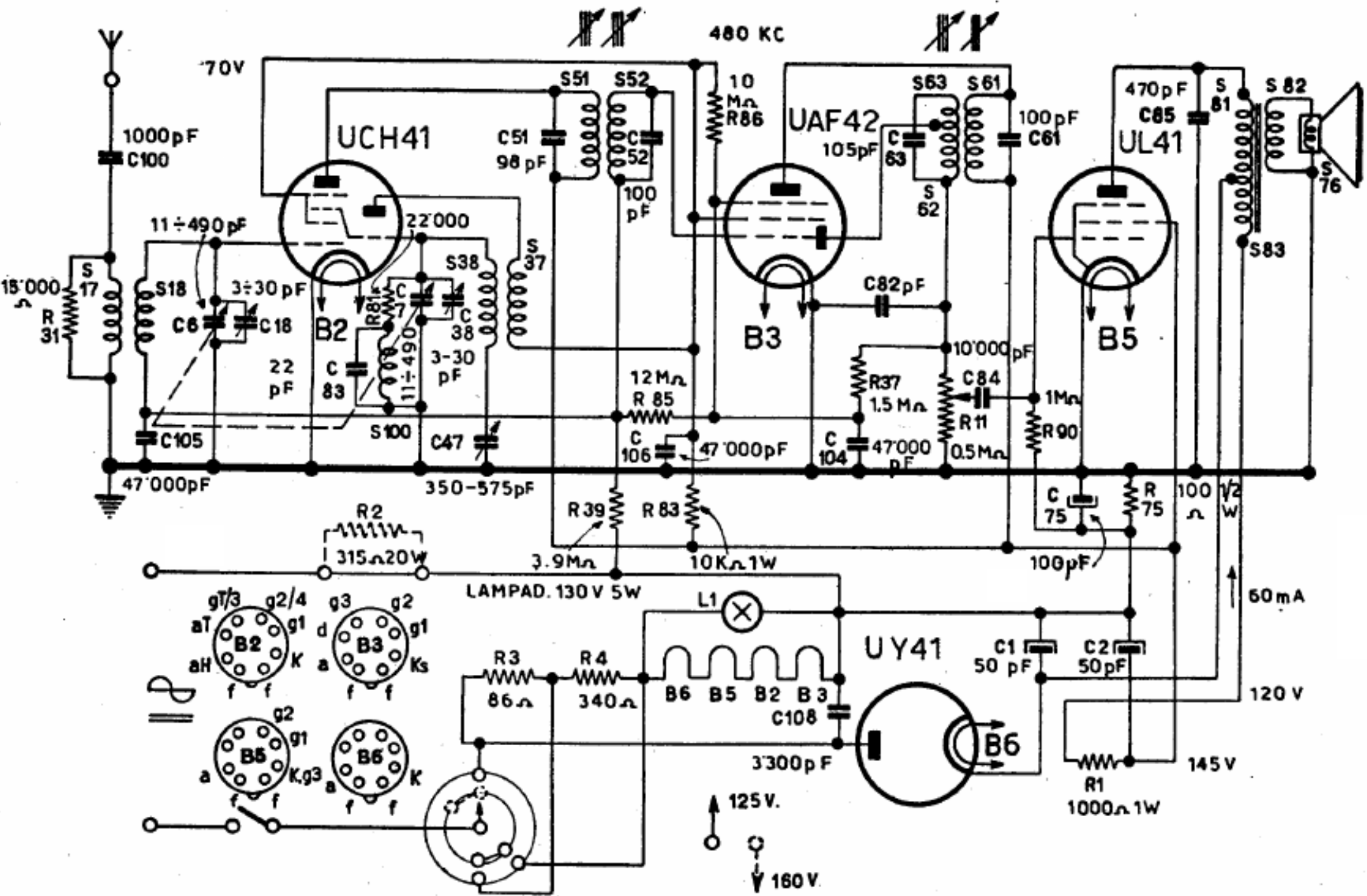
PHILIPS RADIO - Mod. BI 190 U - Gamma onde medie, MF a 468 kc. Placca finale 125 V e 40 mA, schermo 120 V e 7,2 mA. Altre tensioni placche 115 V, schermi 70 V. Corrente totale 60 mA. Consumo 37 W.
